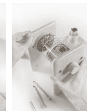
5. Seitenteil abziehen
